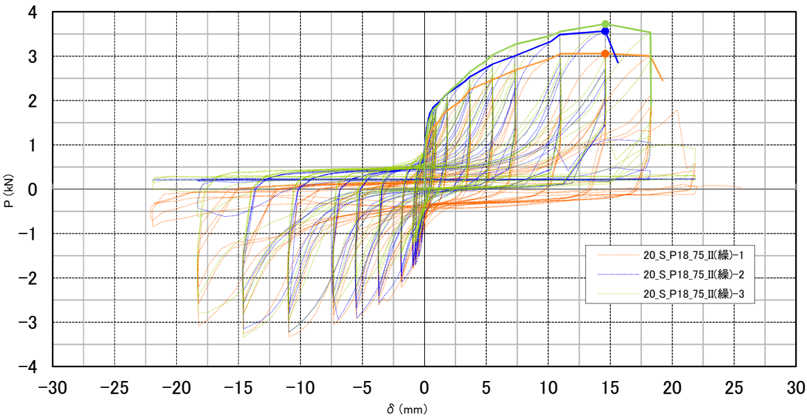
図-45 P-δ 曲線 (試験体相互の比較)
