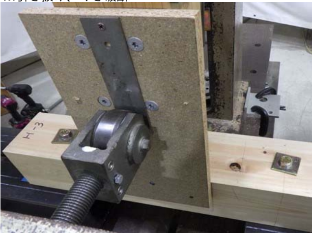
写真-42 「9-S_P18-75_⊥(単) 試験終了後」
