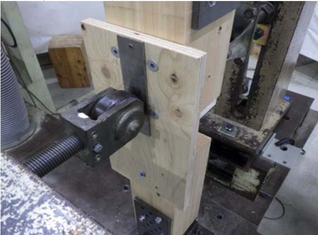
写真-65 「14-S_Wh18-75_II (緑) 試験終了後」
