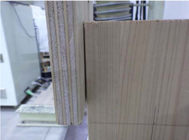
写真-67 「14-S_Wh18-75_II (緑) 試験終了後」
