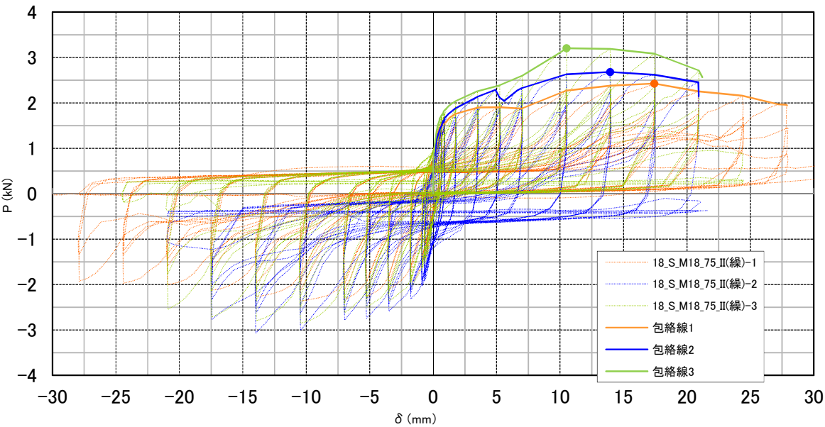
図-41 P-δ 曲線（試験体相互の比較）
