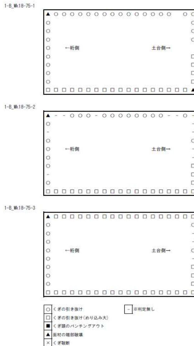
図 4-10 釘の破壊性状一覧
