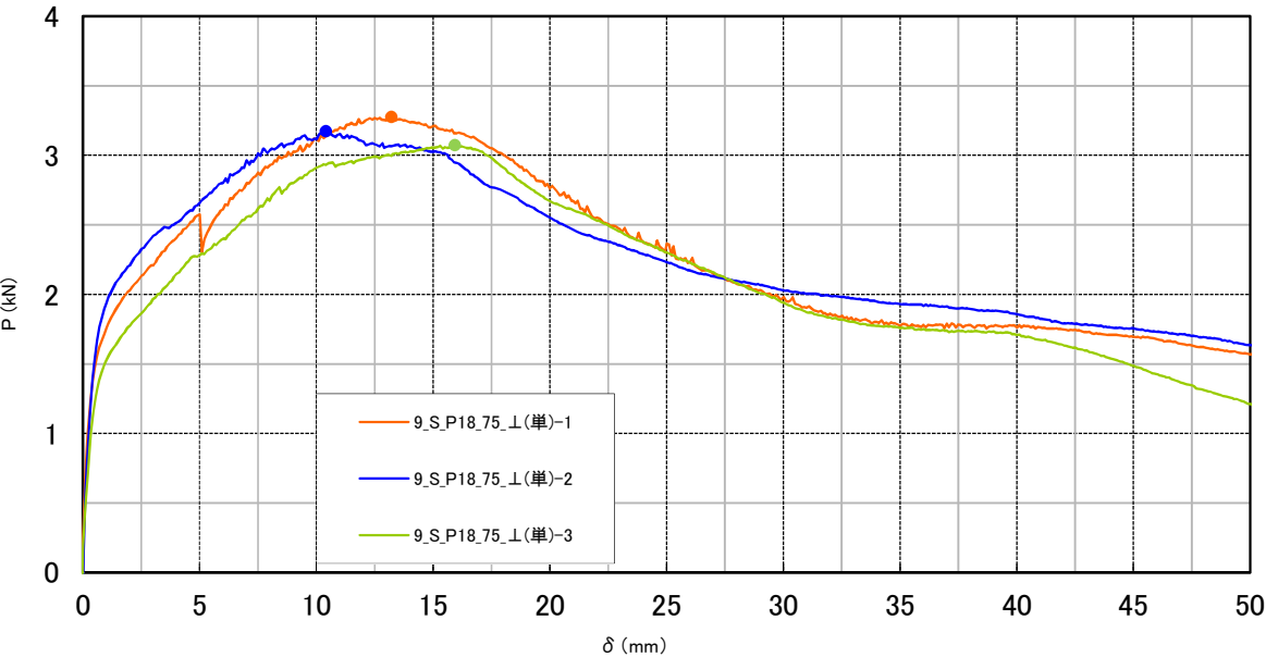
図-23 P-δ 曲線（試験体相互の比較）
