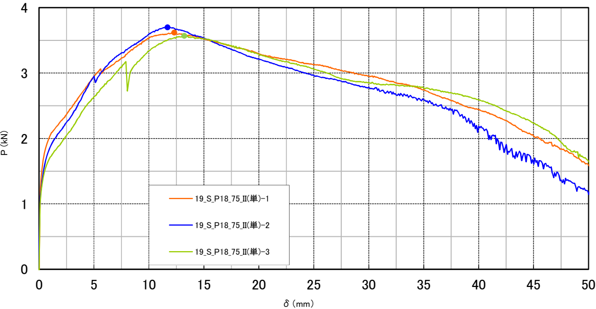
図-43 P-δ 曲線（試験体相互の比較）
