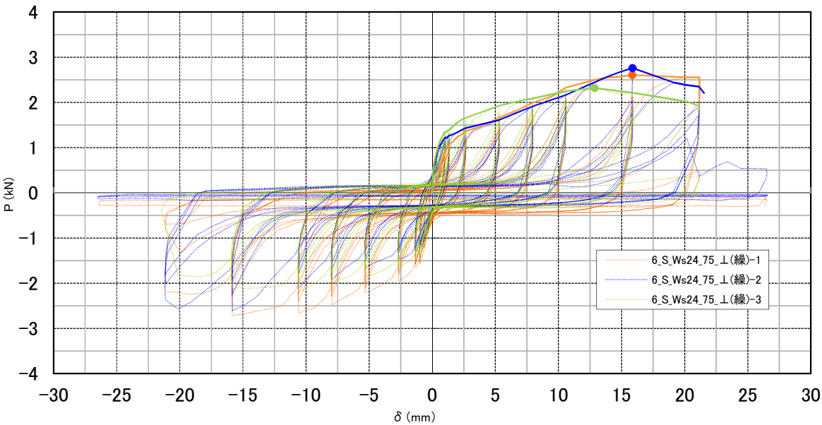
図-17 P-δ 曲線 (試験体相互の比較)
