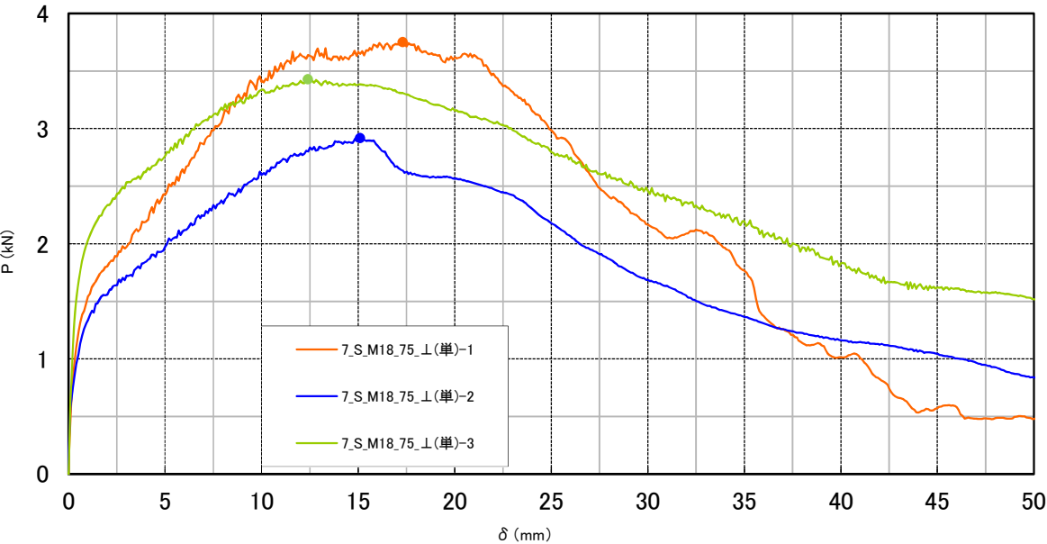
図-19 P-δ 曲線（試験体相互の比較）
