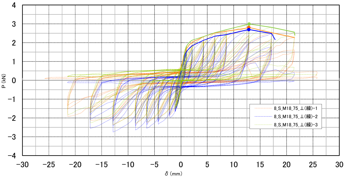
図-21 P-δ 曲線（試験体相互の比較）
