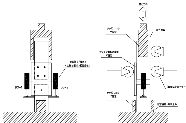
図-5 【繊維平行方向】試験方法 概要図
