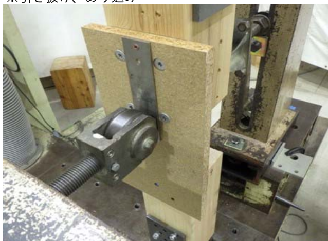
写真-85 「19-S_P18-75_II(単) 試験終了後」
