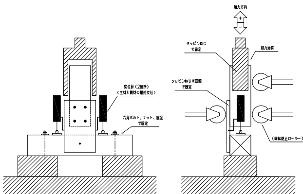
図-4 【繊維直交方向】試験方法 概要図
