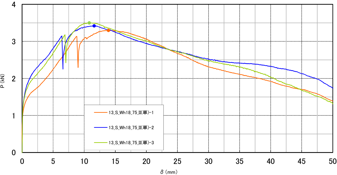
図-31 P-δ 曲線 (試験体相互の比較)
