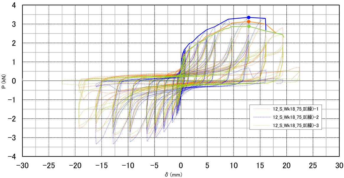
図-29 P-δ 曲線 (試験体相互の比較)
