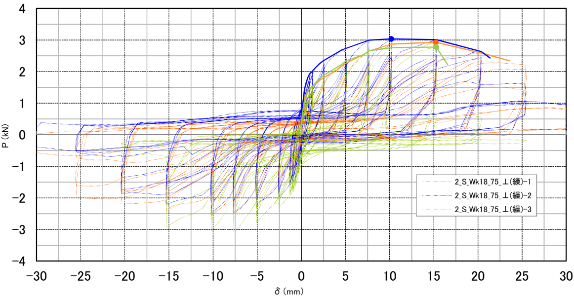
図-9 P-δ 曲線（試験体相互の比較）
