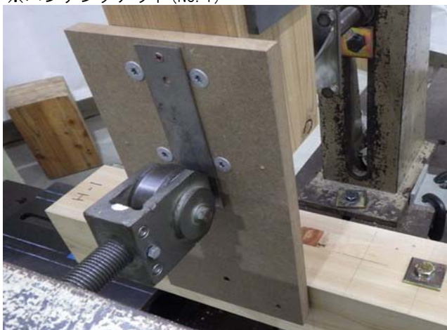
写真-30 「7-S_M18-75_⊥ (単) 試験終了後」
