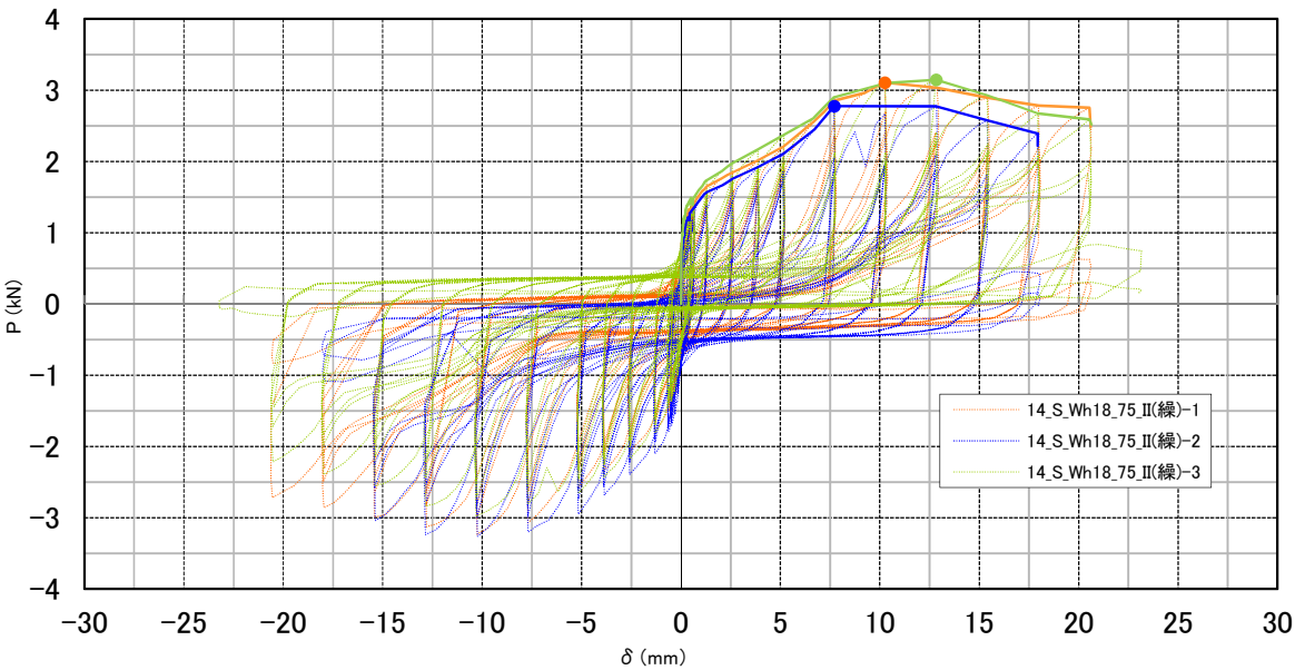
図-33 P-δ 曲線 (試験体相互の比較)
