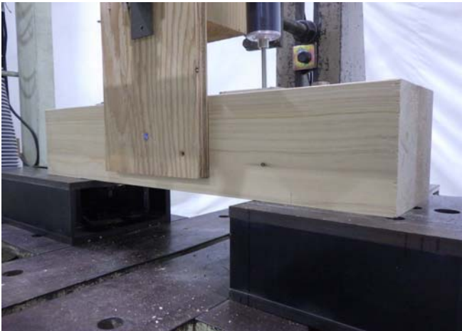
写真-1 【繊維直交方向】試験体設置状況
