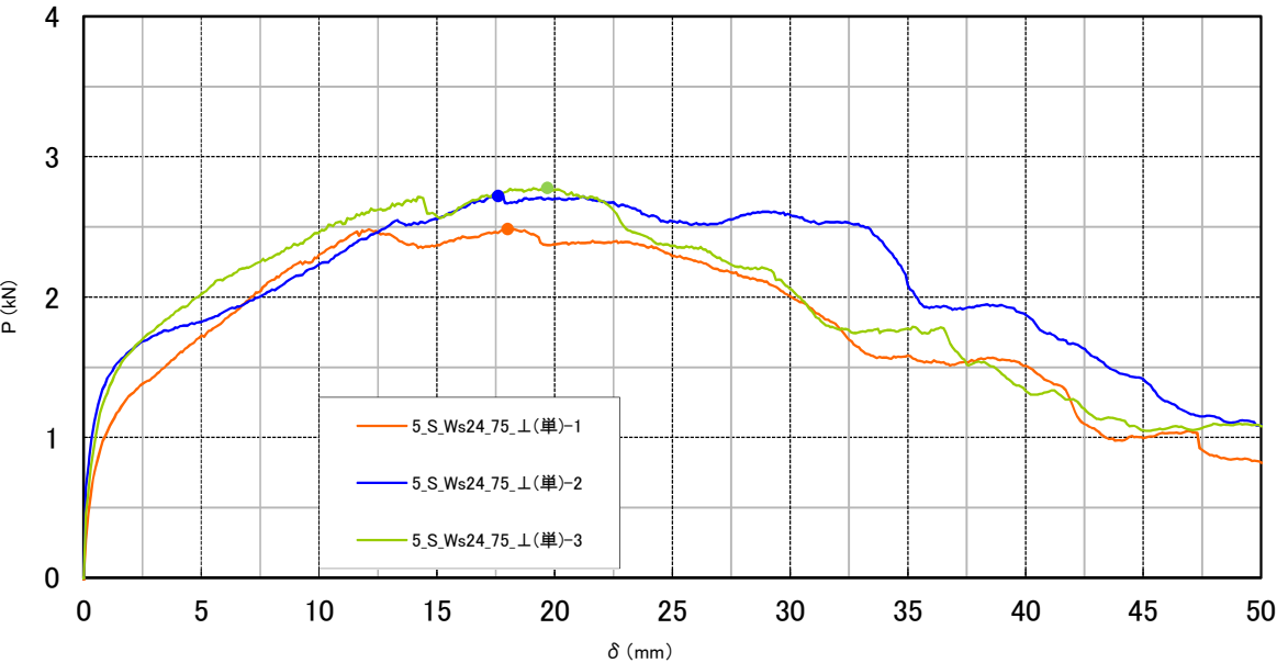
図-15 P-δ 曲線（試験体相互の比較）
