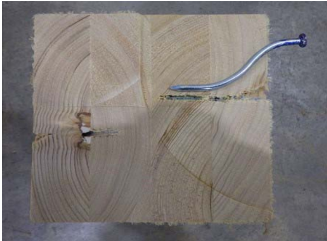
写真-17 「3-S_Wh18-75_⊥(単) 解体後」
