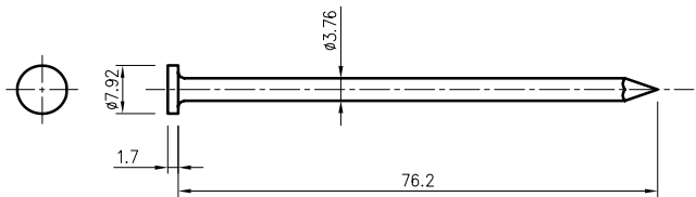
図-3 製品図
