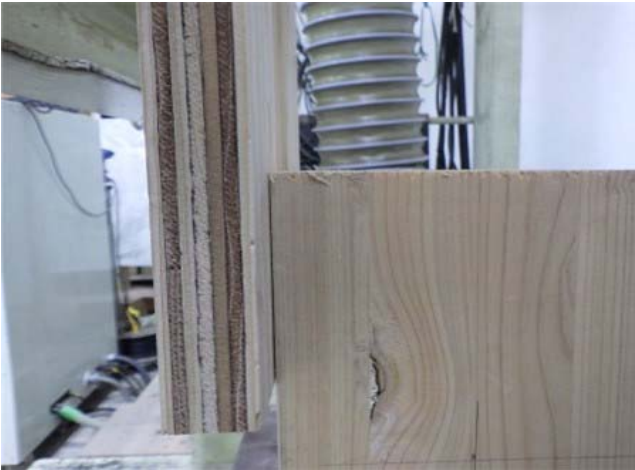
写真-75 「16-S_Ws24-75_II(緑) 試験終了後」
