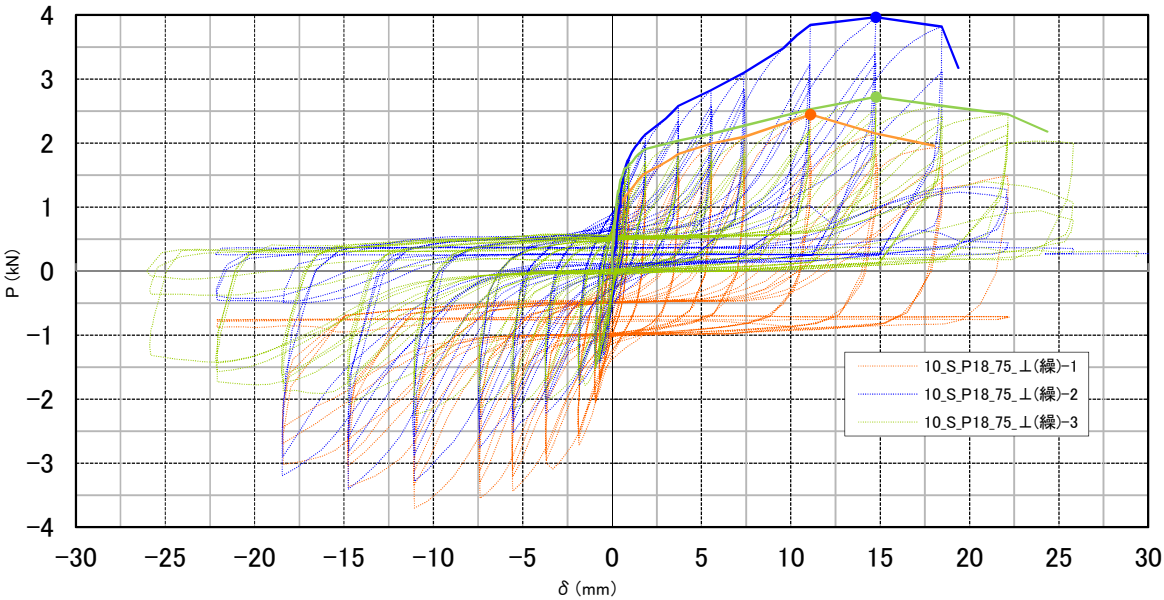
図-25 P-δ 曲線（試験体相互の比較）
