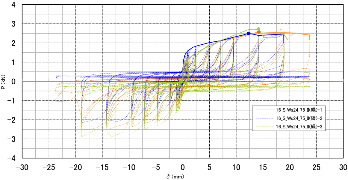
図-37 P-δ 曲線 (試験体相互の比較)
