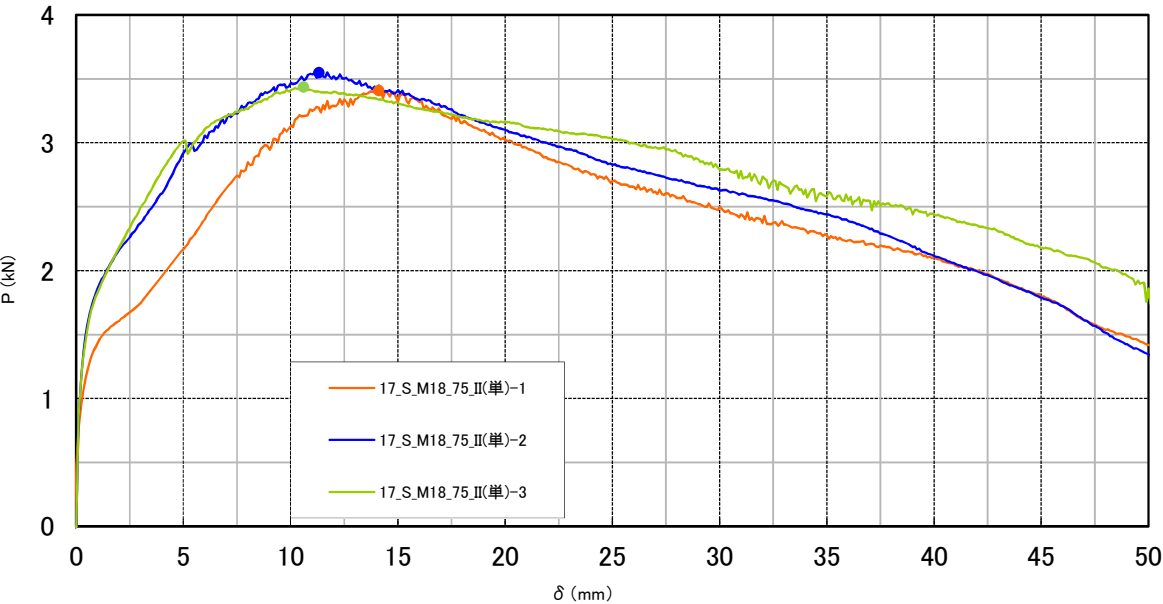
図-39 P-δ 曲線（試験体相互の比較）
