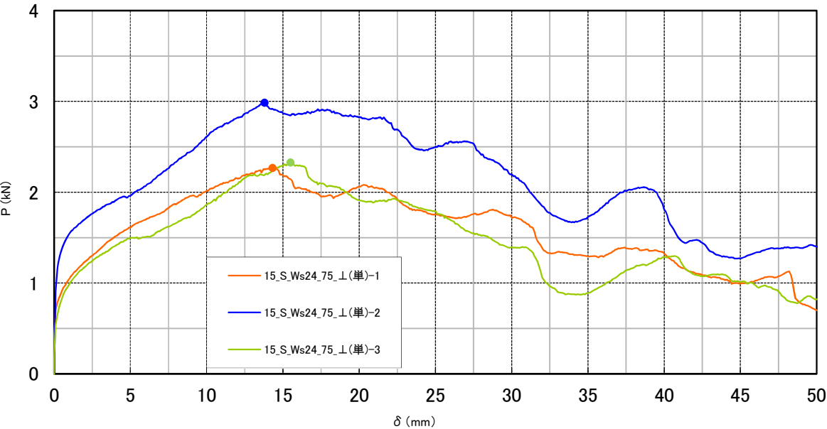
図-35 P-δ 曲線 (試験体相互の比較)
