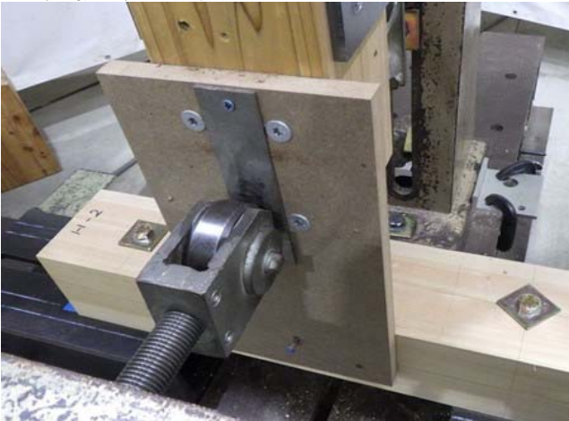
写真-38 「8-S_M18-75_⊥(繰) 試験終了後」
