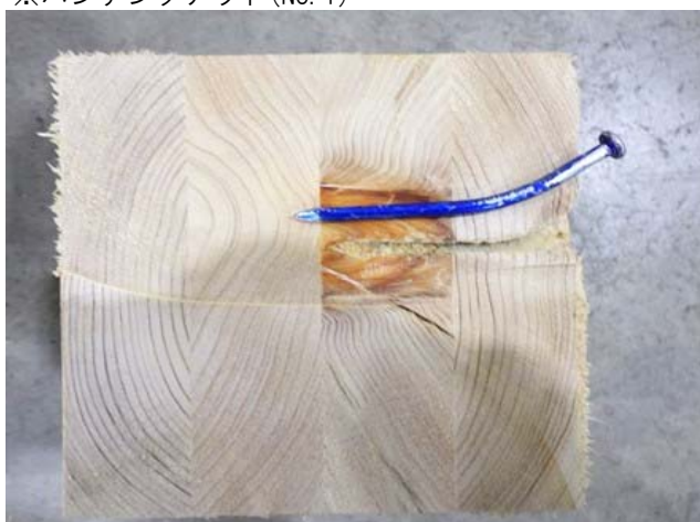
写真-33 「7-S_M18-75_⊥ (単) 解体後」
