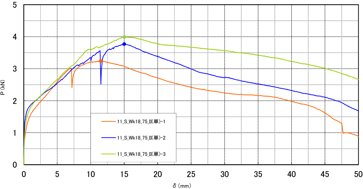
図-27 P-δ 曲線（試験体相互の比較）
